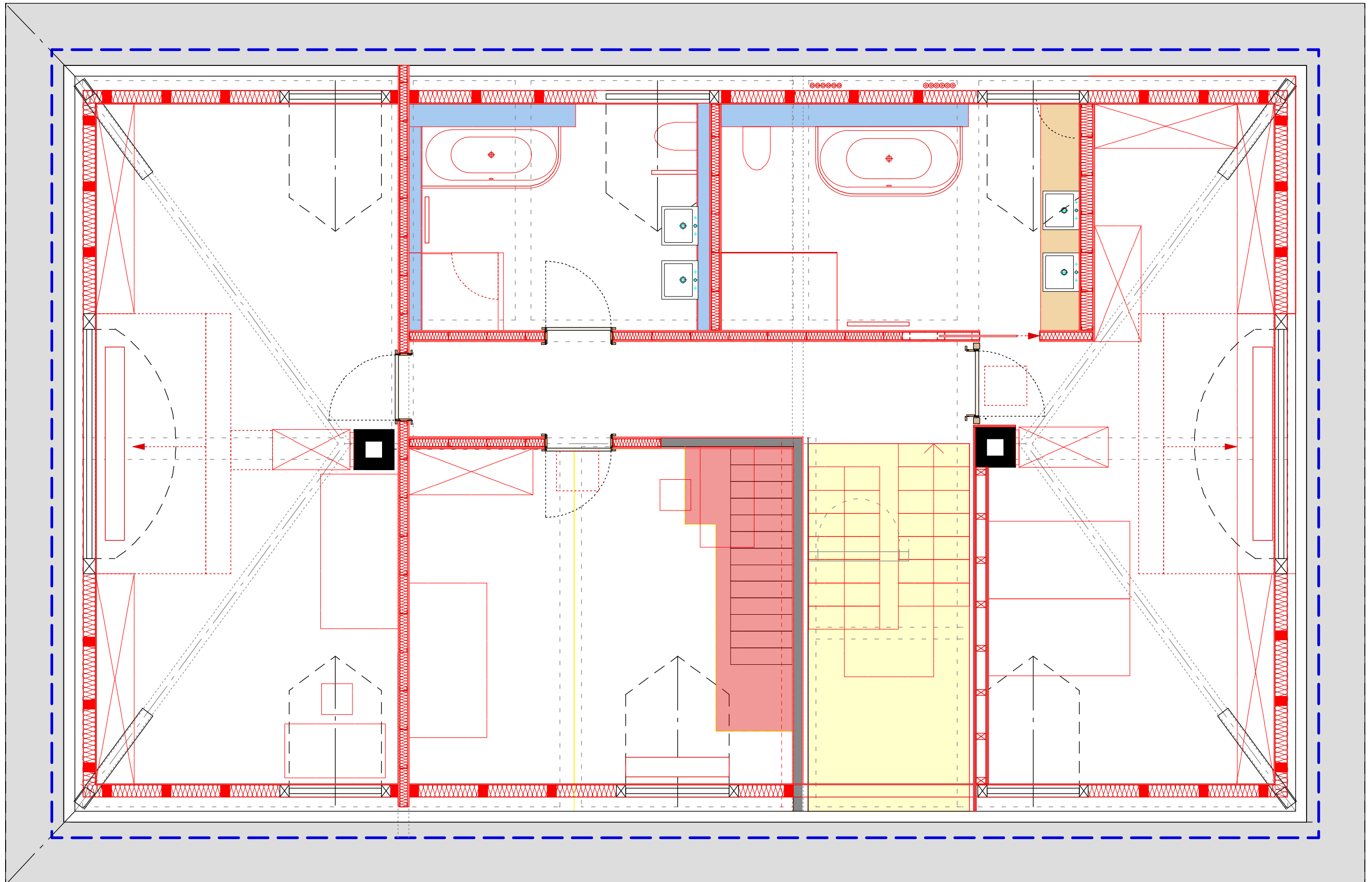
Ausbau Dachgeschoss Grundriss DG 1/50
